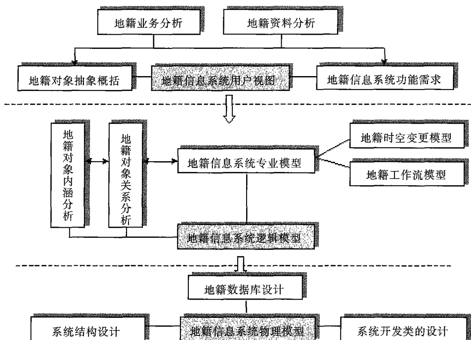
图3 基于面向对象方法的地籍信息系统的分析设计过程
