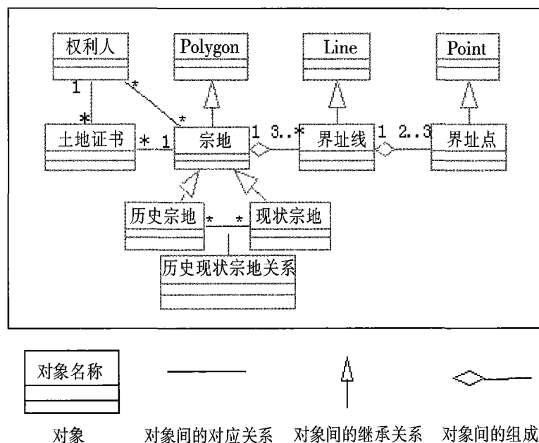
图4 地籍间对象逻辑模型图
