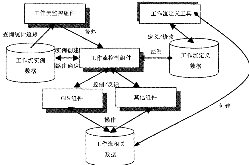
图6 GIS 组件和工作流组件组成的地籍信息系统结构
